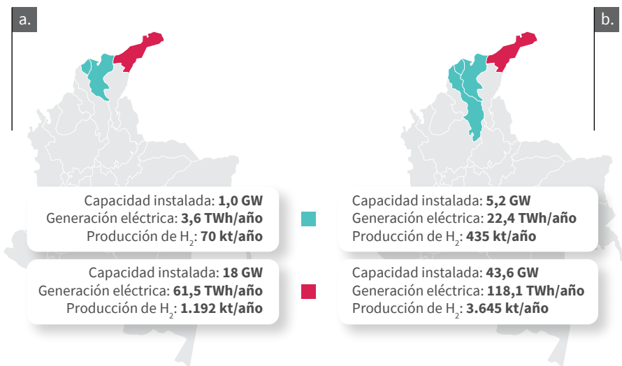
FIGURA 7. POTENCIAL EÓLICO (A) COSTA ADENTRO Y (B) COSTA AFUERA PARA LA INSTALACIÓN, GENERACIÓN ELÉCTRICA Y PRODUCCIÓN DE HIDRÓGENO
