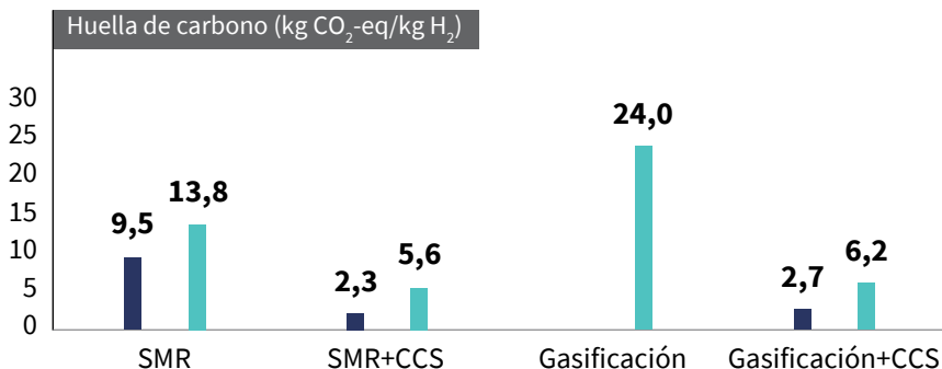
FIGURA 14. HUELLA DE CARBONO PARA LOS DIFERENTES MÉTODOS DE PRODUCCIÓN DE HIDRÓGENO GRIS Y AZUL A PARTIR DE RECURSOS FÓSILES.
